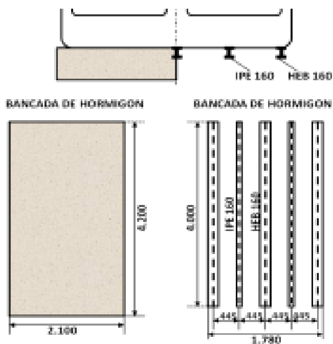
Fig. 17 (EWK 900)
