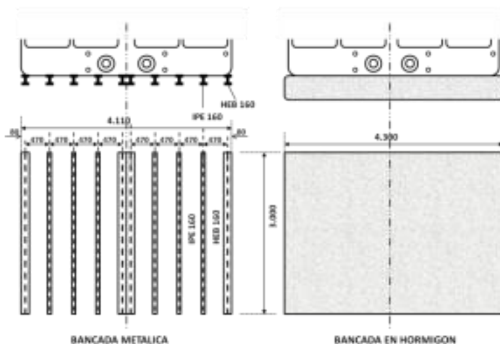
Fig. 18 (EWK 1260)
